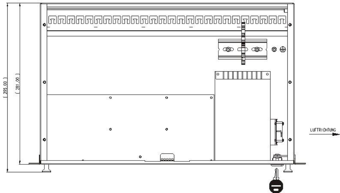
DRAUSICHT OHNE DECKEL
